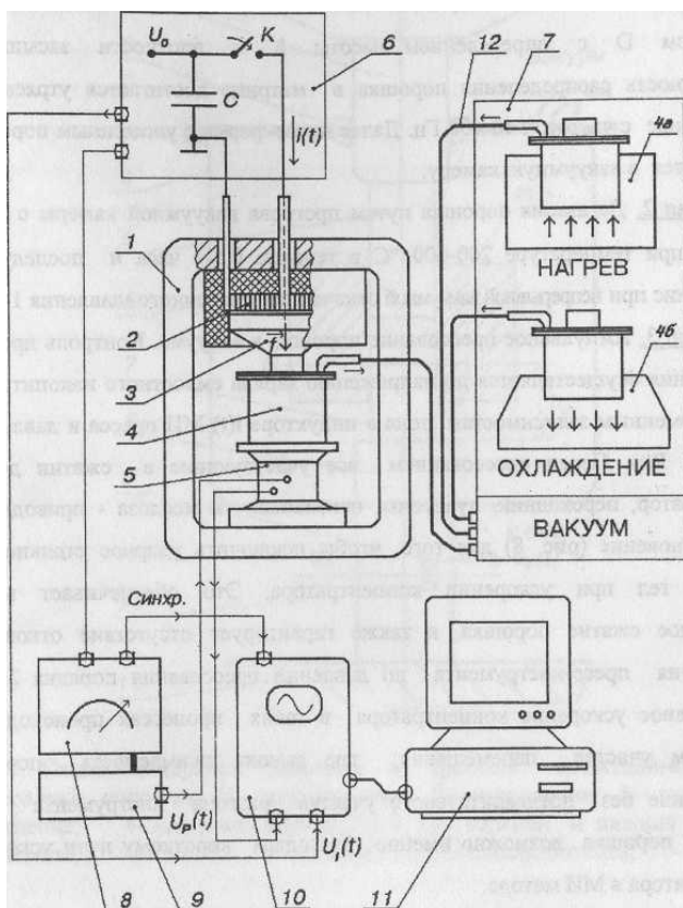
Рис. 7. Блок схема установки для МИ прессования порошков:
