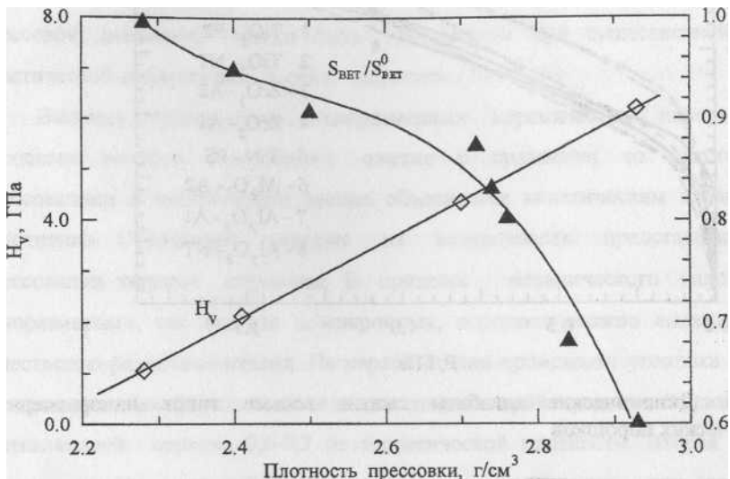
Рис. 4. Микротвердость и относительная поверхность прессовок нанопорошка из \text{Al}_2\text{O}_3 в зависимости от их плотности
